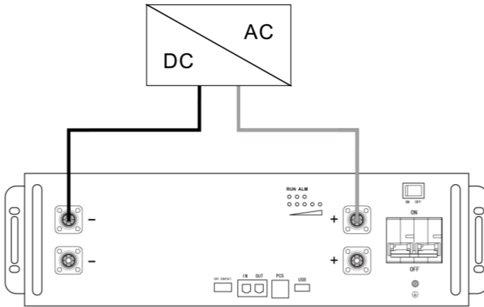
Abbildung 5-2: Einzelbatterieanschluss
